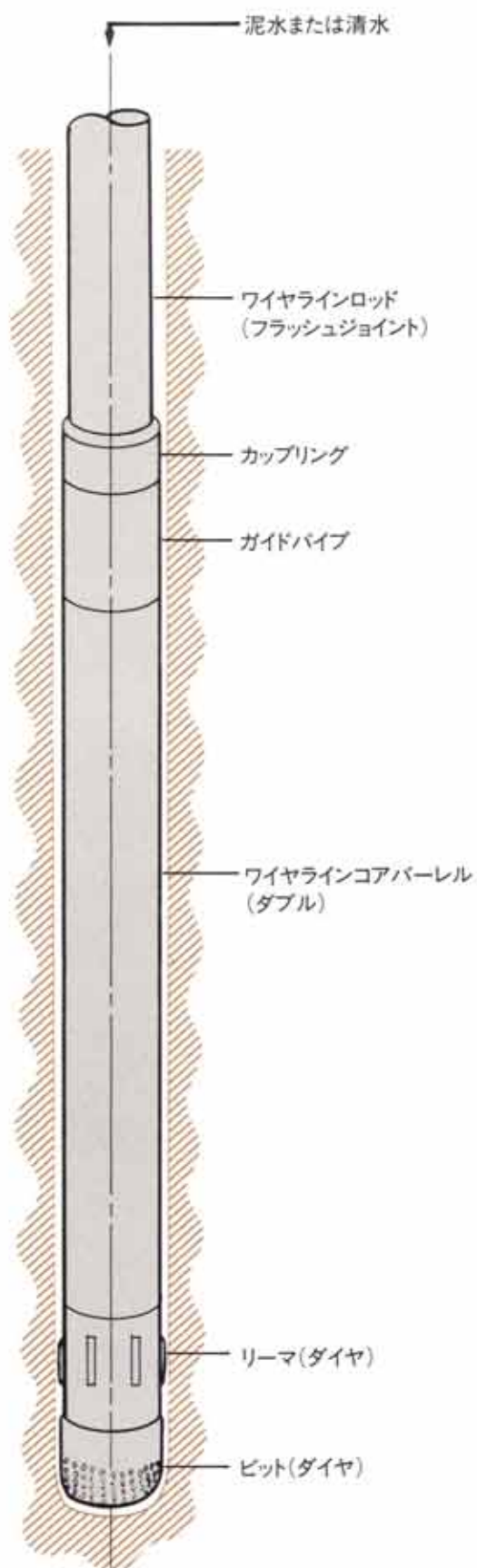
(2) ワイヤライン工法ツールス
