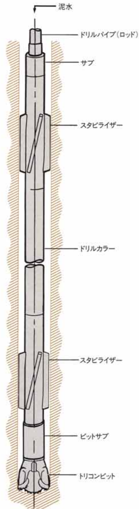
(3) ノンコアリング工法ツールス
