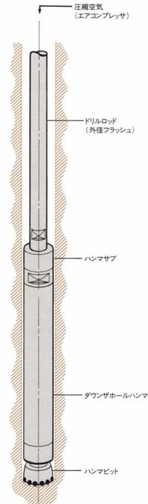
(4) ダウンザホールハンマ工法ツールス
