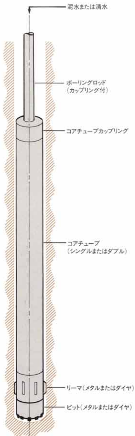
(1) 普通工法ツールス
